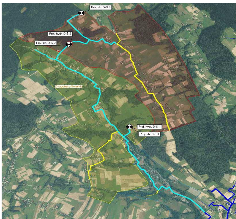
Zdjęcie nr 13 „Poprawa gospodarki wodno-ściekowej na terenie gminy Podegrodzie”-„Przebudowa i rozbudowa sieci wodociągowej w kierunku miejscowości Długoteka-Świerkla oraz przebudowa sieci wodociągowej Budowa kanalizacji sanitarnej w m. Gostwica” cz. I.
